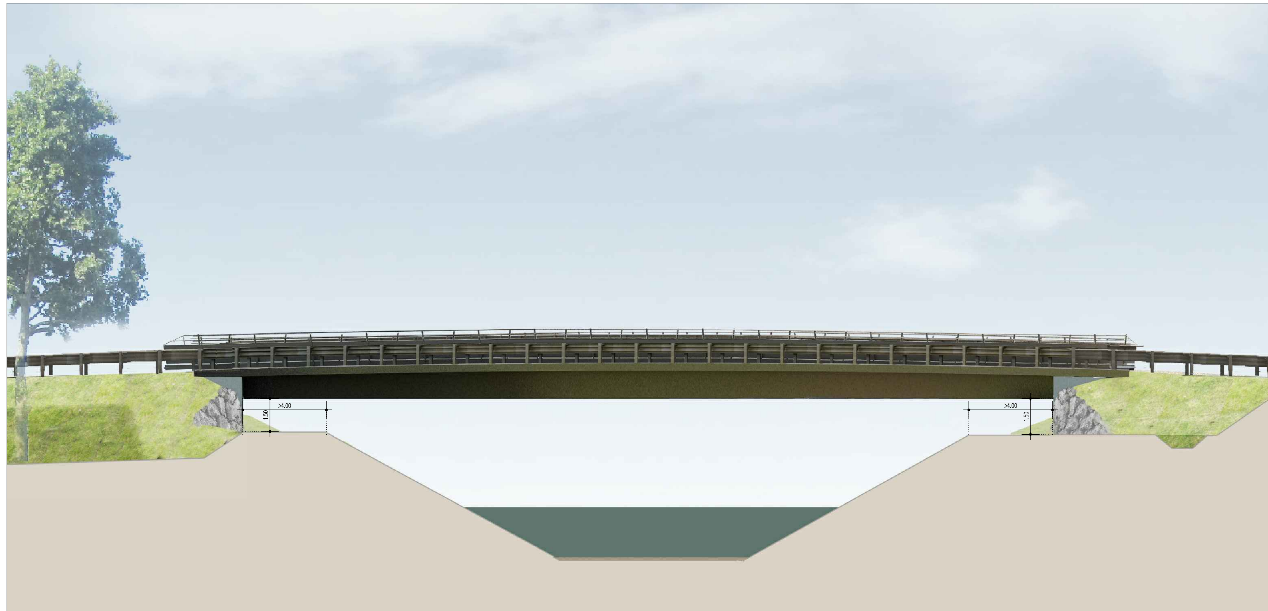
PROSPETTO EST - 1:100
