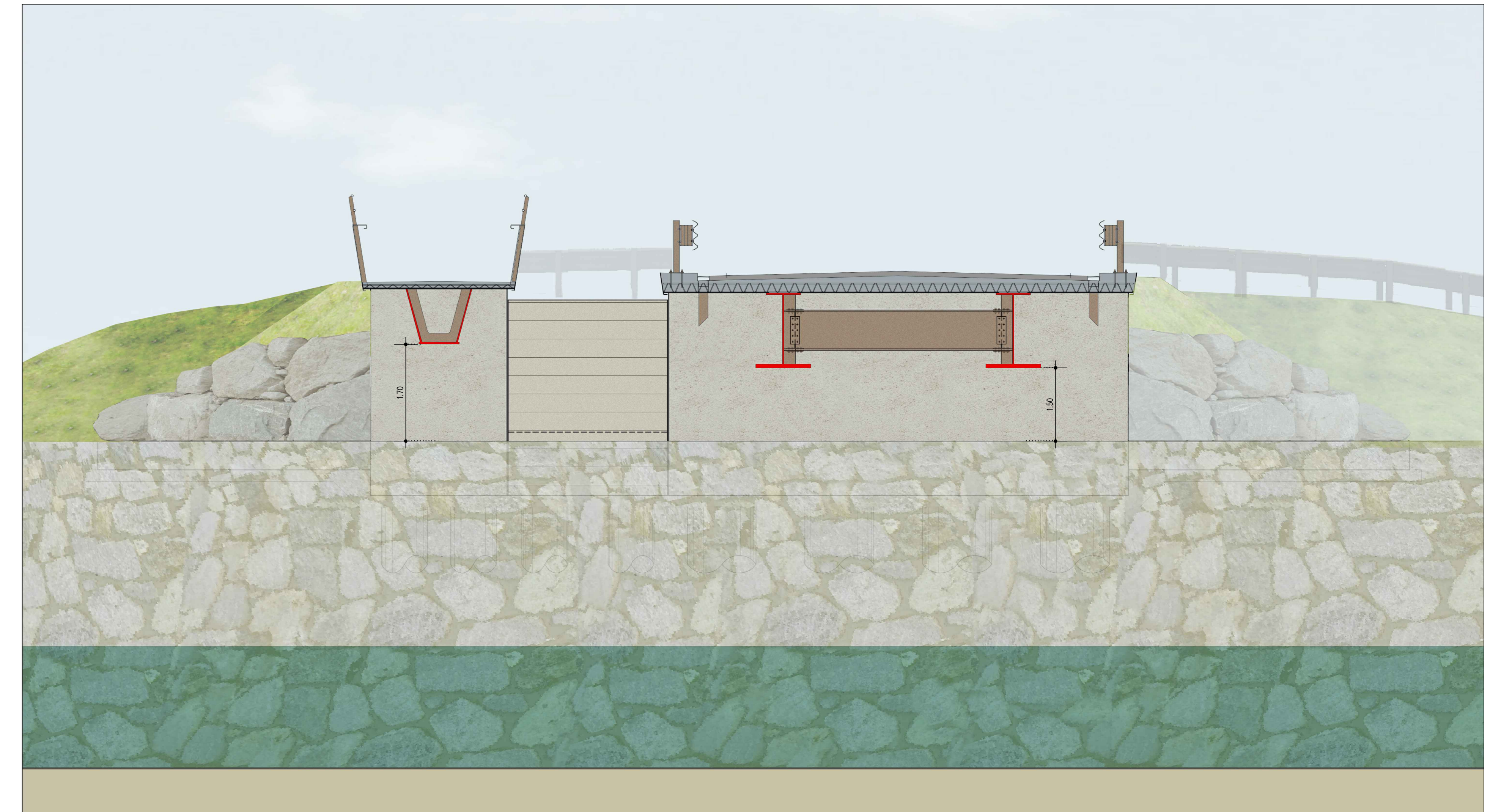
SEZIONE IMPALCATI E PROSPETTO SPALLA NORD - 1:50
