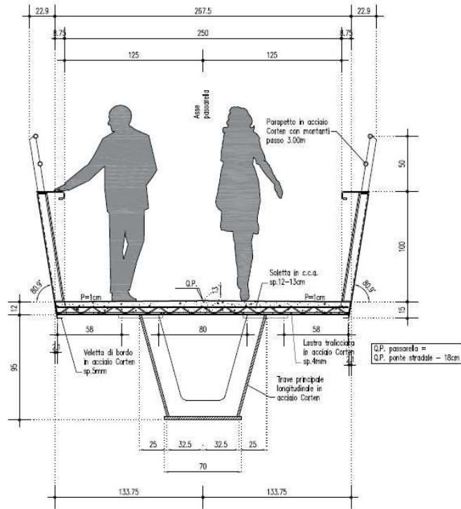
PASSARELLA CICLOPEDONALE
