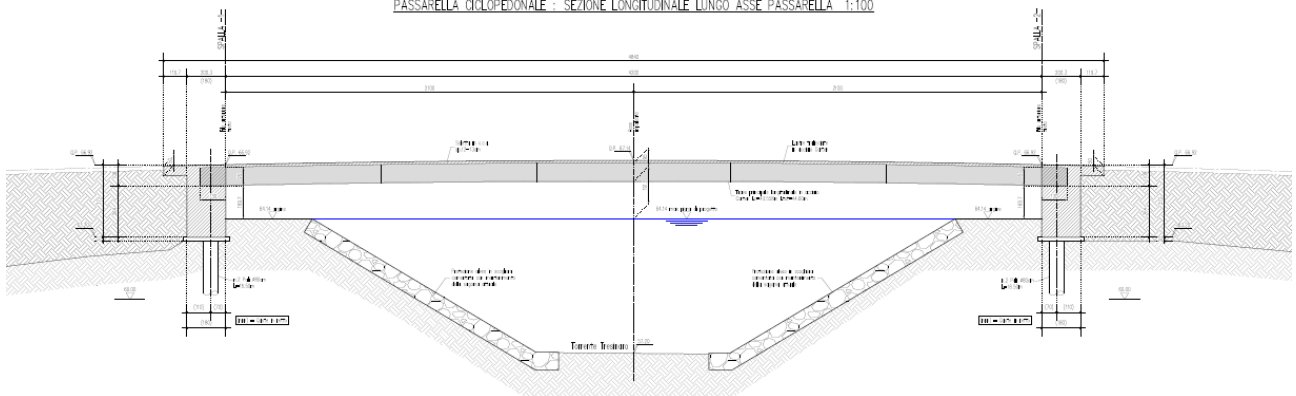
PASSARELLA CICLOPEDONALE - SEZIONE LONGITUDINALE LUNGO ASSE PASSARELLA 1:100
