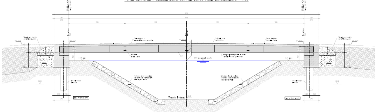
PONTE STRADALE : SEZIONE LONGITUDINALE LUNGO ASSE TRACCIAMENTO 1:100
